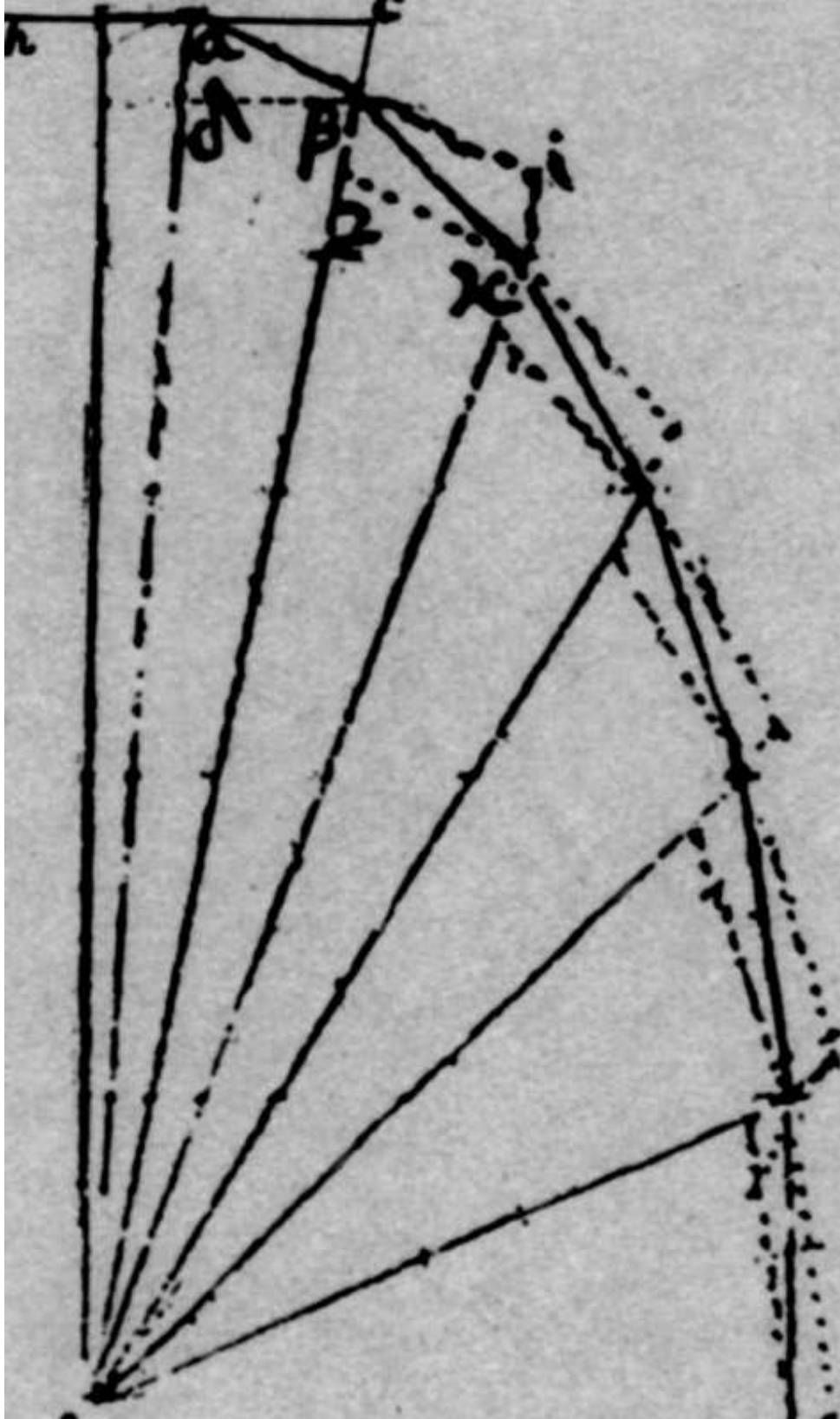
Figure 2 Diagramme partiel de Hooke en septembre 1685 pour une approximation discrète d'une orbite elliptique.
